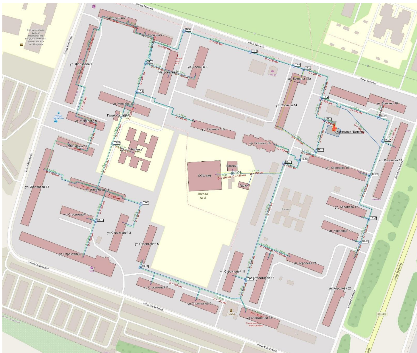
Схема 6. - Зона действия котельной 18 МВт (Есенина)
