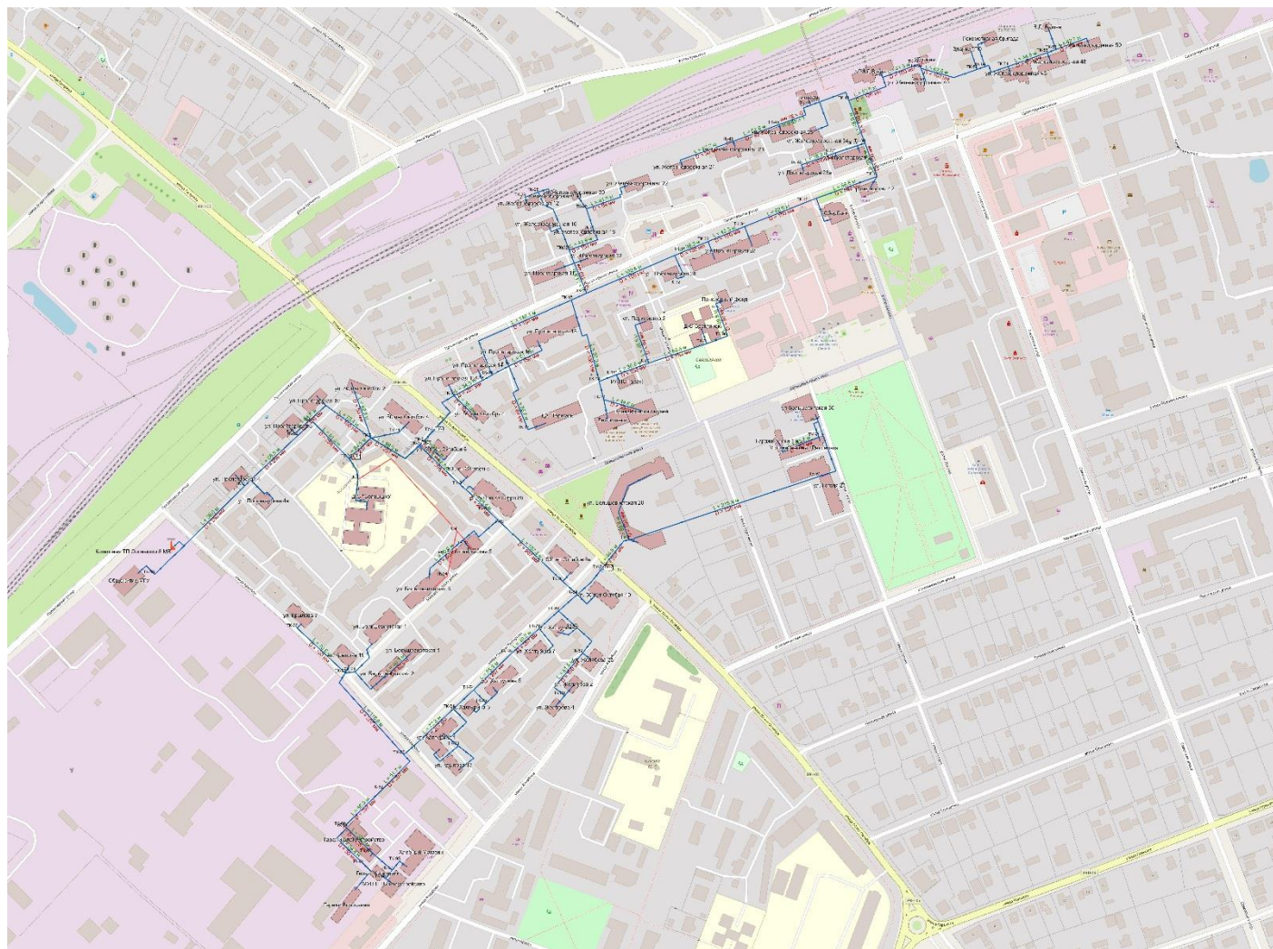
Схема 9. - Зона действия котельной 8МВт (Солнышко)
