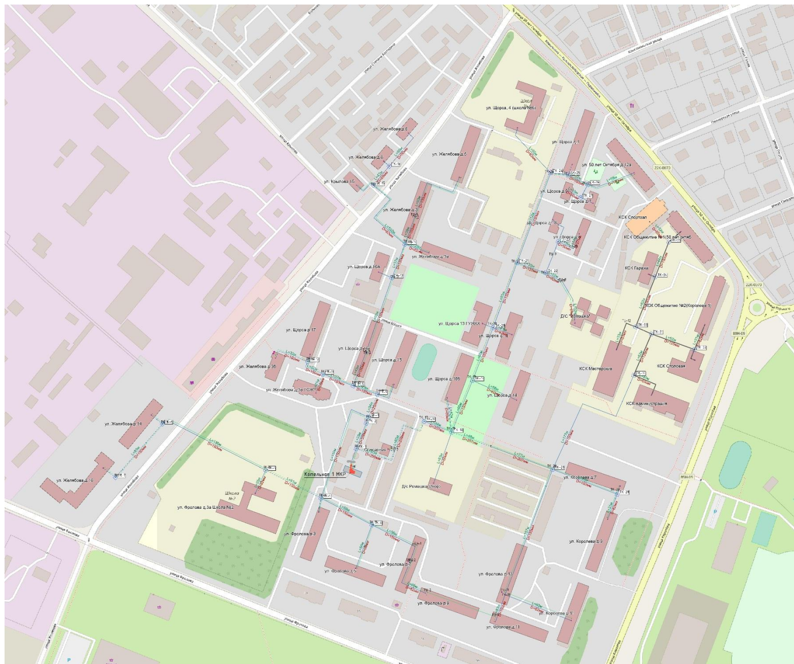
Схема 1. - Зона действия котельной 12МВт (1-й микрорайон г. Ковылкино)
