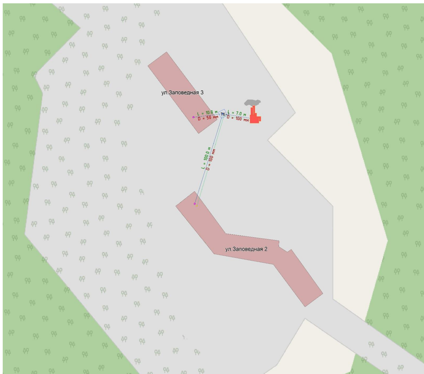
Схема 11. - Зона действия котельной по ул. Заповедная, 5
