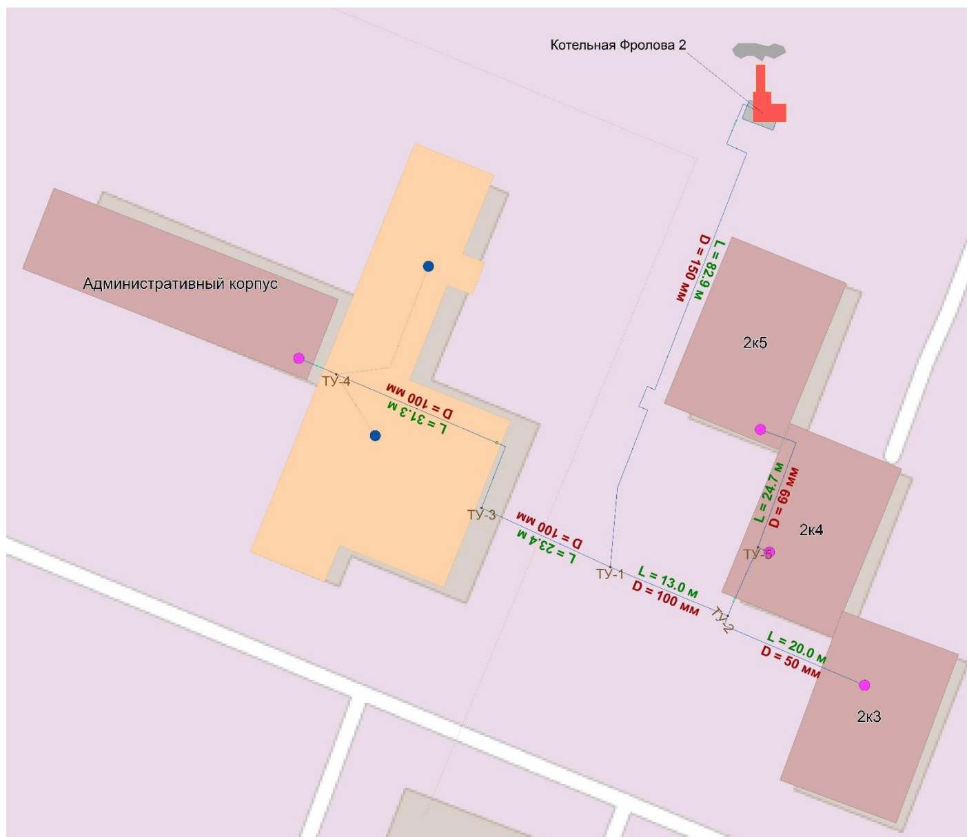
Схема 15. - Зона действия котельной ул. Фролова, д. 2А г. Ковылкино
