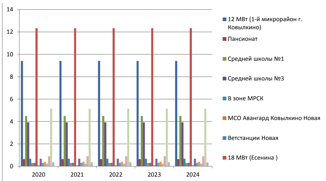
Рисунок 4.1. - Прогнозируемые к 2024 г. приросты тепловых нагрузок в зонах действия энергоисточников.
