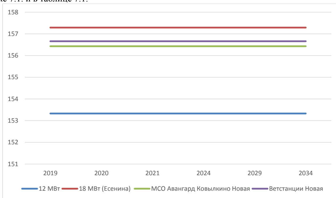
Рисунок 7.1. Динамика НУР топлива на период 2020-2034 г.г.
